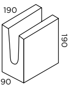
10.12 Lintel 5.3kg 360 per pallet 1908kg pallet weight
